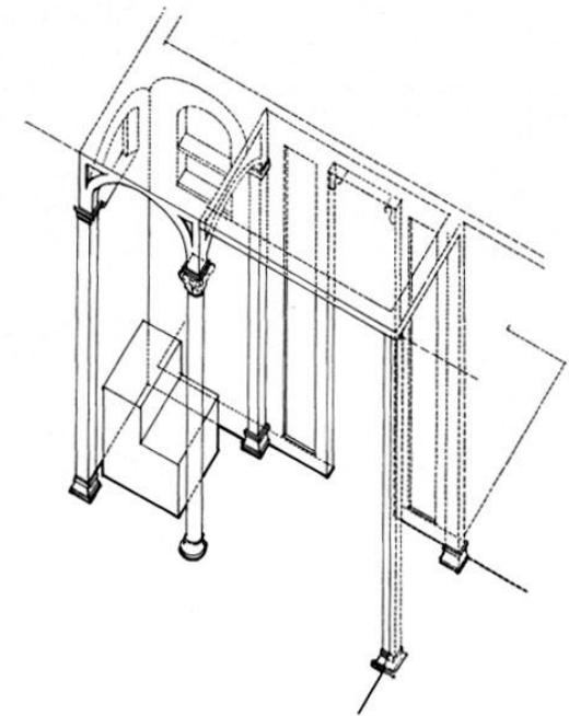
La Collegiata di Castiglione Olona - Varese Parete del presbiterio E - Storie di Santo Stefano "Chiamata in giudizio" - Paolo Schiavo Pianta - prospetto e restituzione assonometrica della struttura architettonica CLASSE 3 BSL LICEO ARTISTICO "A.FRATTINI" VARESE - SPERIMENTAZIONE LEONARDO - INDIRIZZO BENI CULTURALI A.S. 2000/2001
